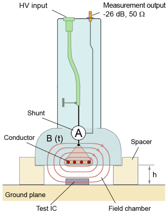
P1202-4 EFT/burst H-field source
