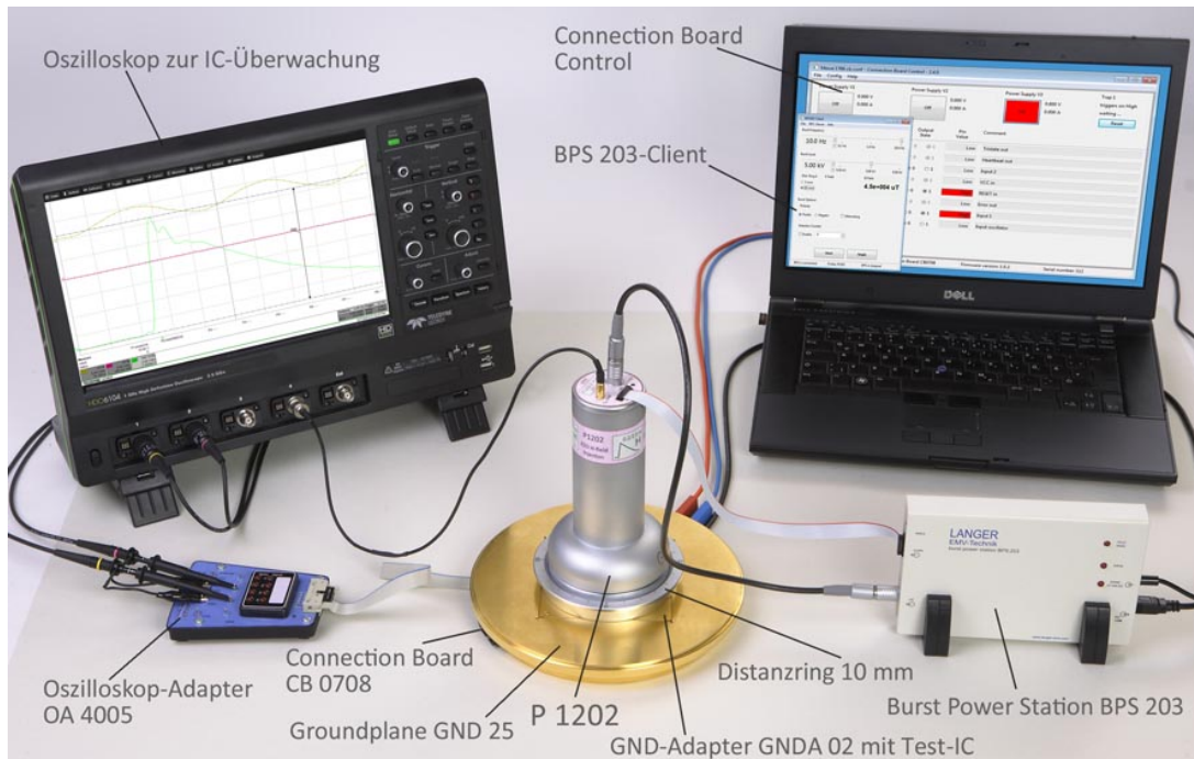
Messplatz mit P1202 L-ESD Magnetfeldquelle Langer Puls 0,2/2,5 ns
