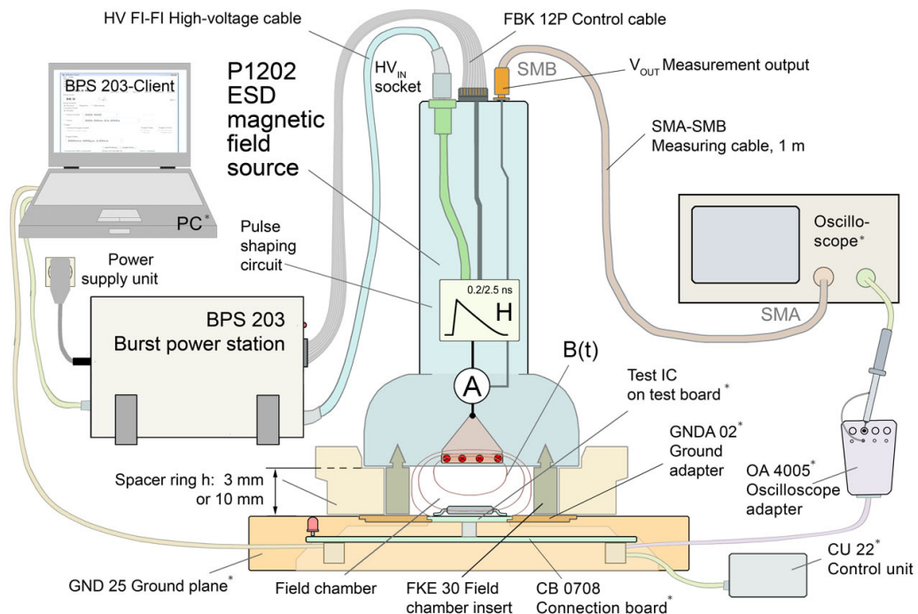
Messanordnung mit P1202 L-ESD (Die mit * gekennzeichneten Geräte sind nicht im Lieferumfang enthalten.)
