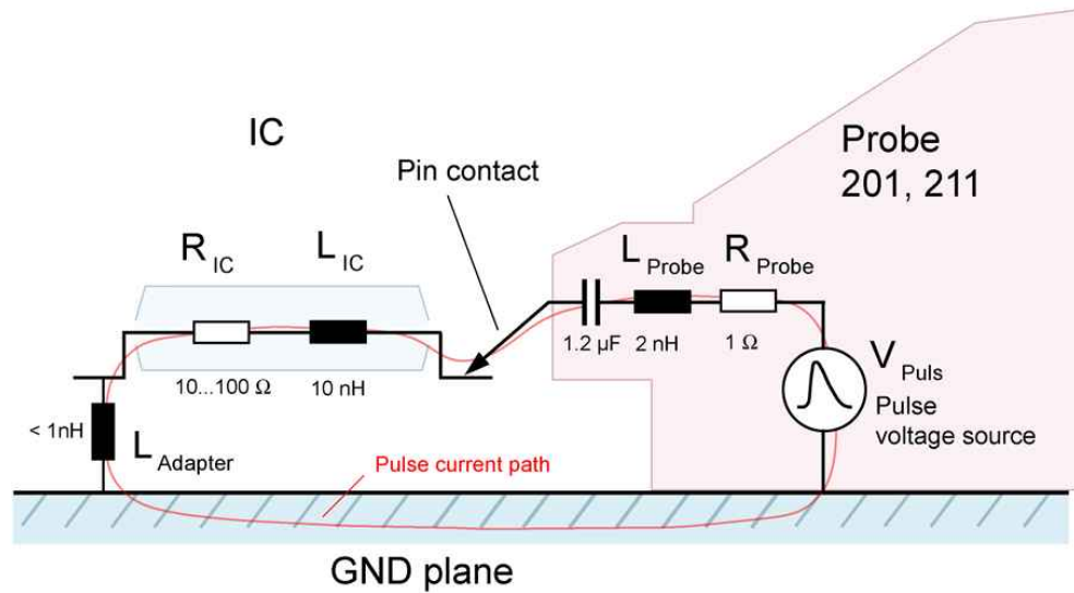
Ersatzschaltbild
