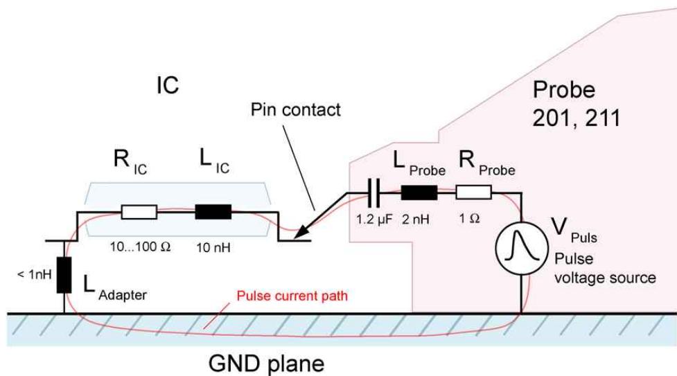
Ersatzschaltbild
