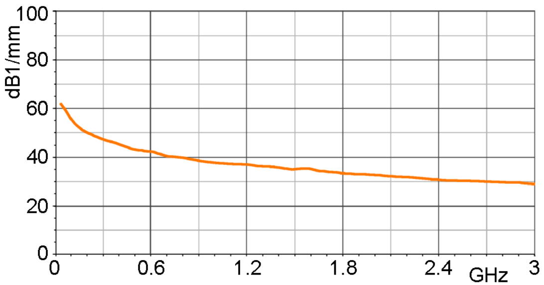
Korrekturkurve E-Feld [dBµV/mm] / [dBµV]
