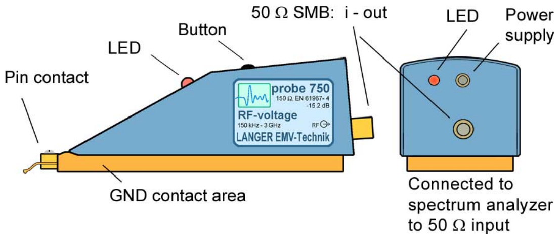
Aufbau Ansicht 01
