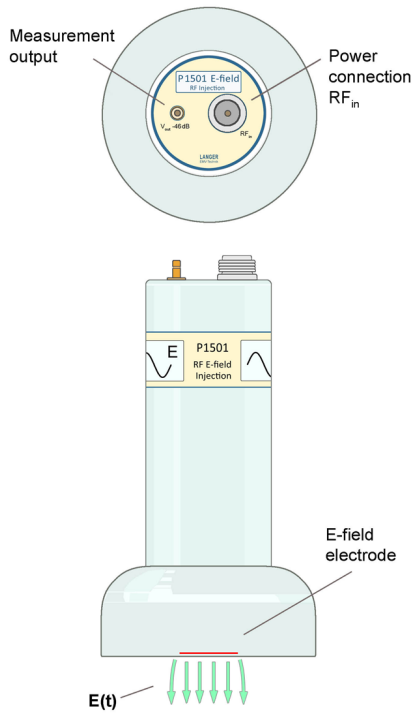
安装视图 01
