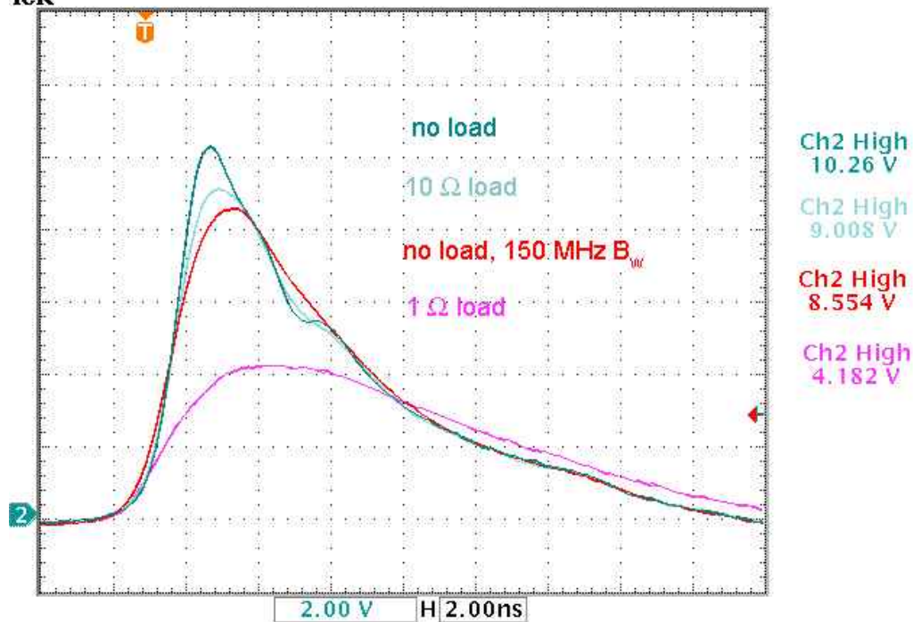
脉冲形状 (实测)
