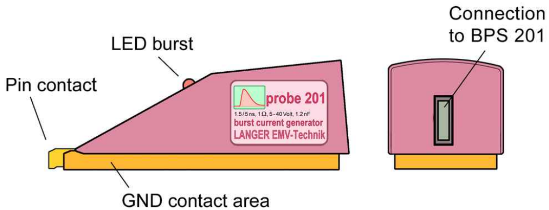
安装视图 01
