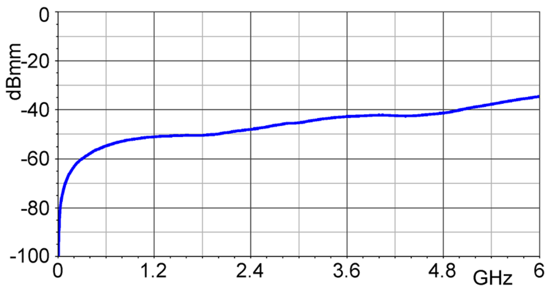
频率特性 [dBμV] / [dBμA/m]
