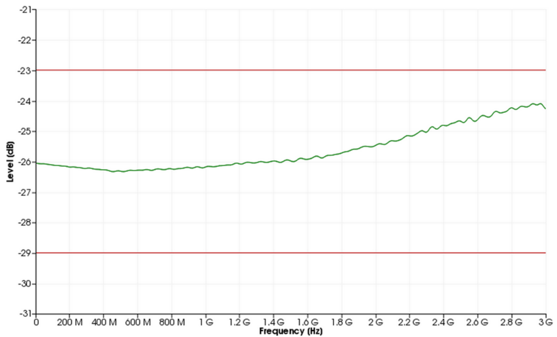
频率特性
