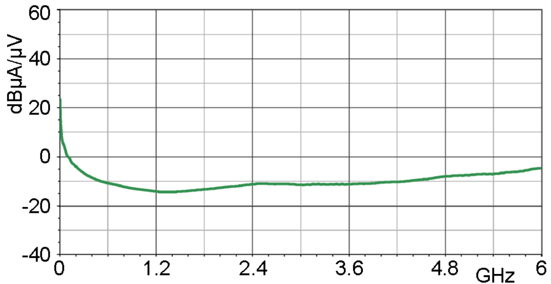
电流校正曲线 [dBμA] / [dBμV]
